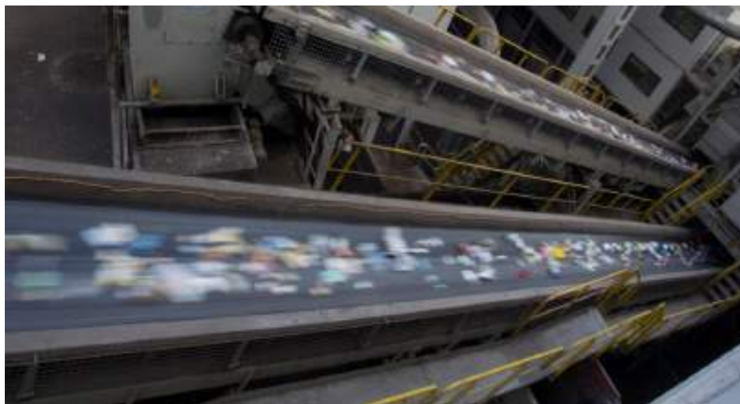
Recuperación de plástico mediante separadores ópticos
