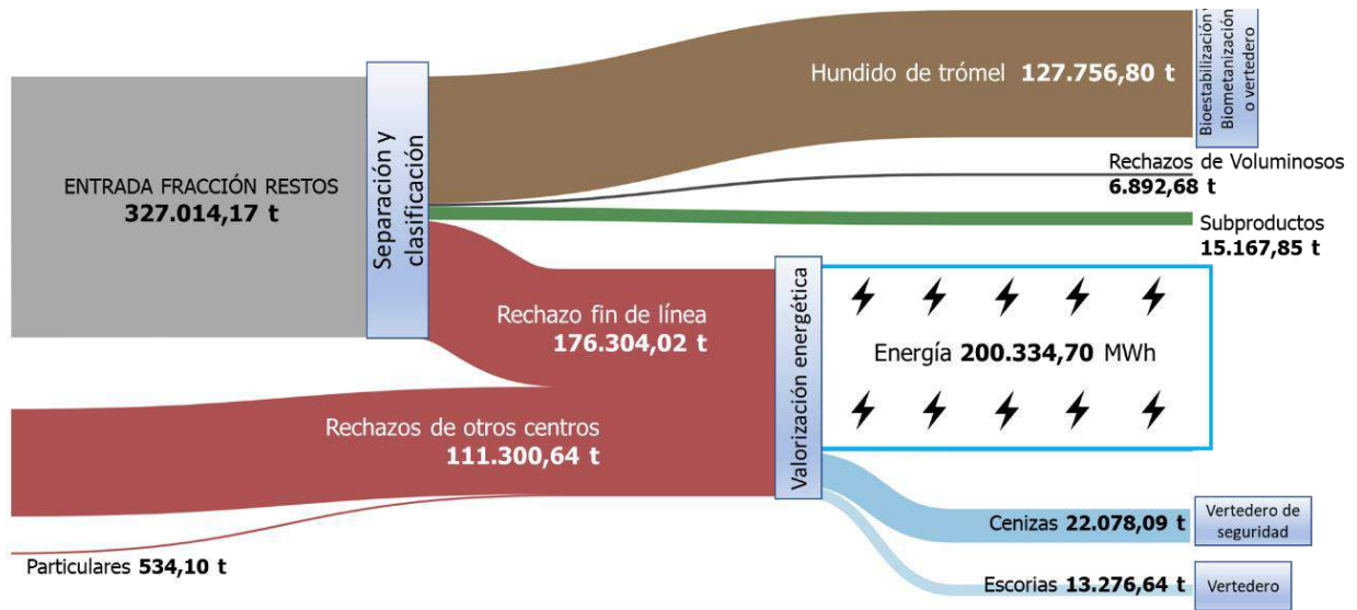
Gráfico 5.2. Gestión de residuos en Las Lomas en el año 2022
