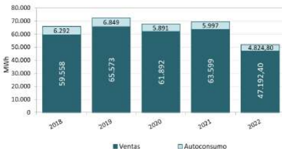
Gráfico 6.1. Destino de la electricidad generada en La Galiana (2018-2022)
