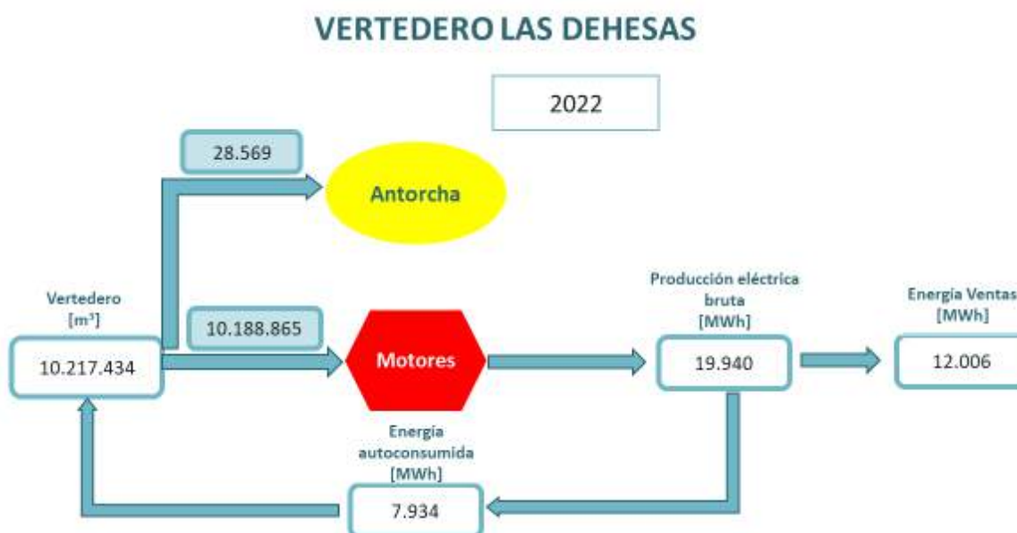
Gráfico 4.4. Biogás extraído del vertedero y producción de energía eléctrica (2022)
