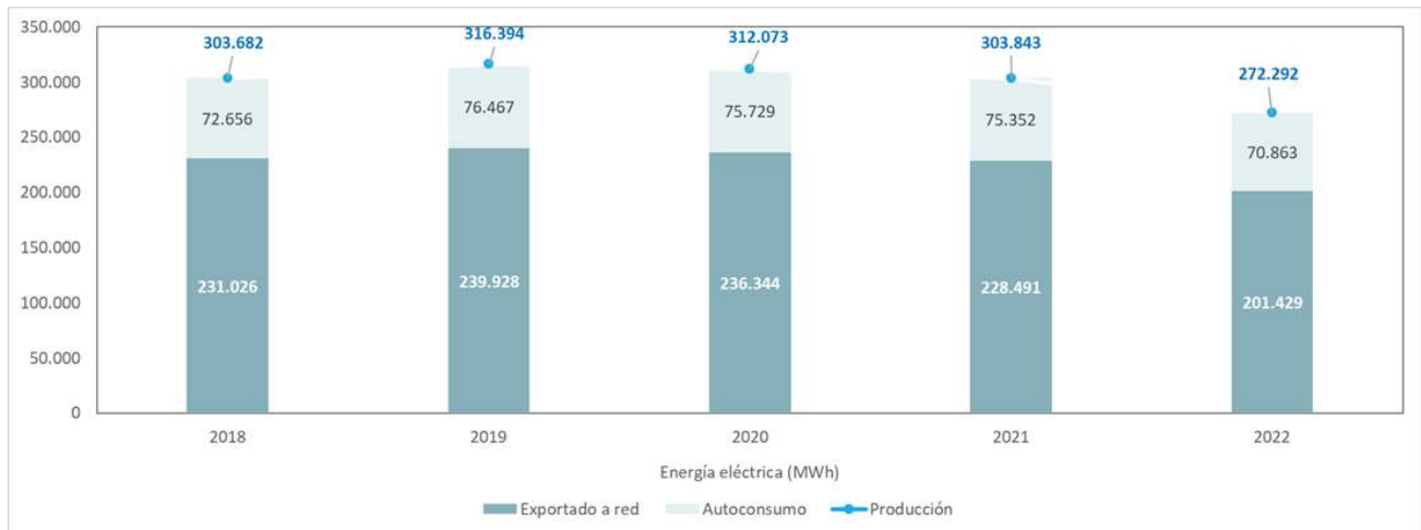
Gráfico 1.9. Generación y destino de la energía eléctrica en el PTV (2018-2022)
