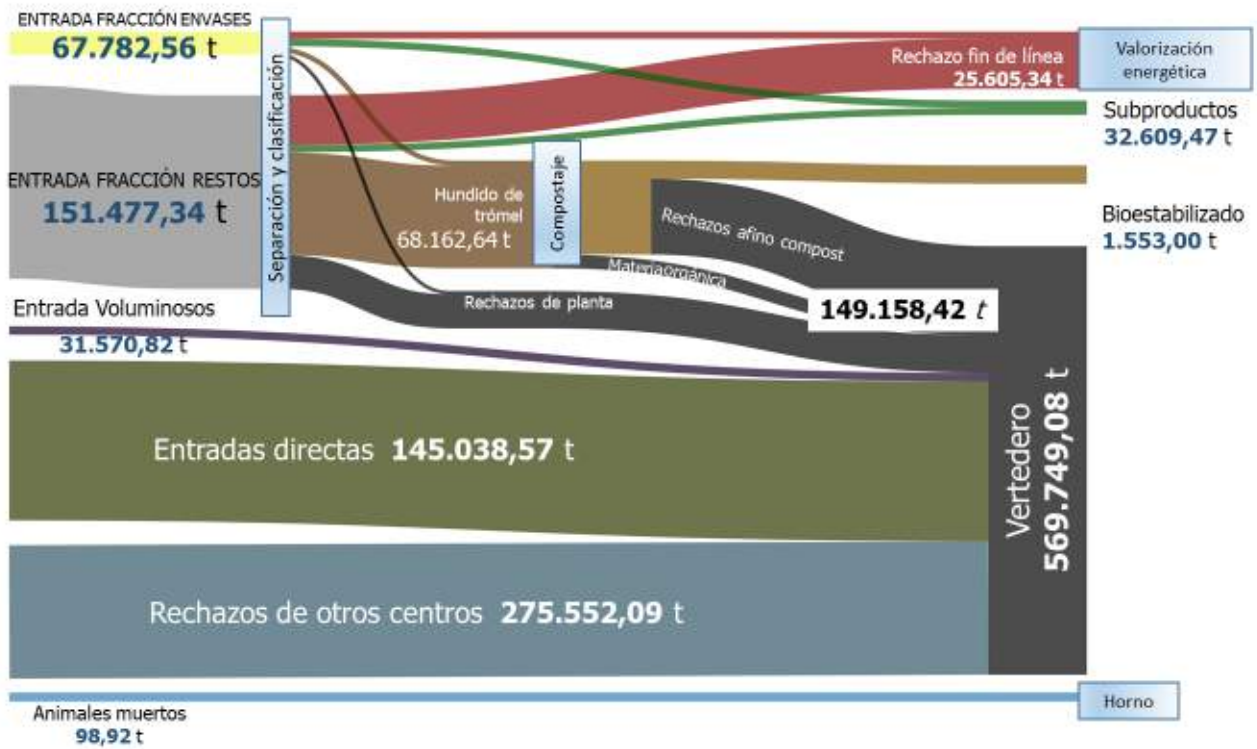
Gráfico 4.5. Esquema gestión de residuos en el centro Las Dehesas en 2022
