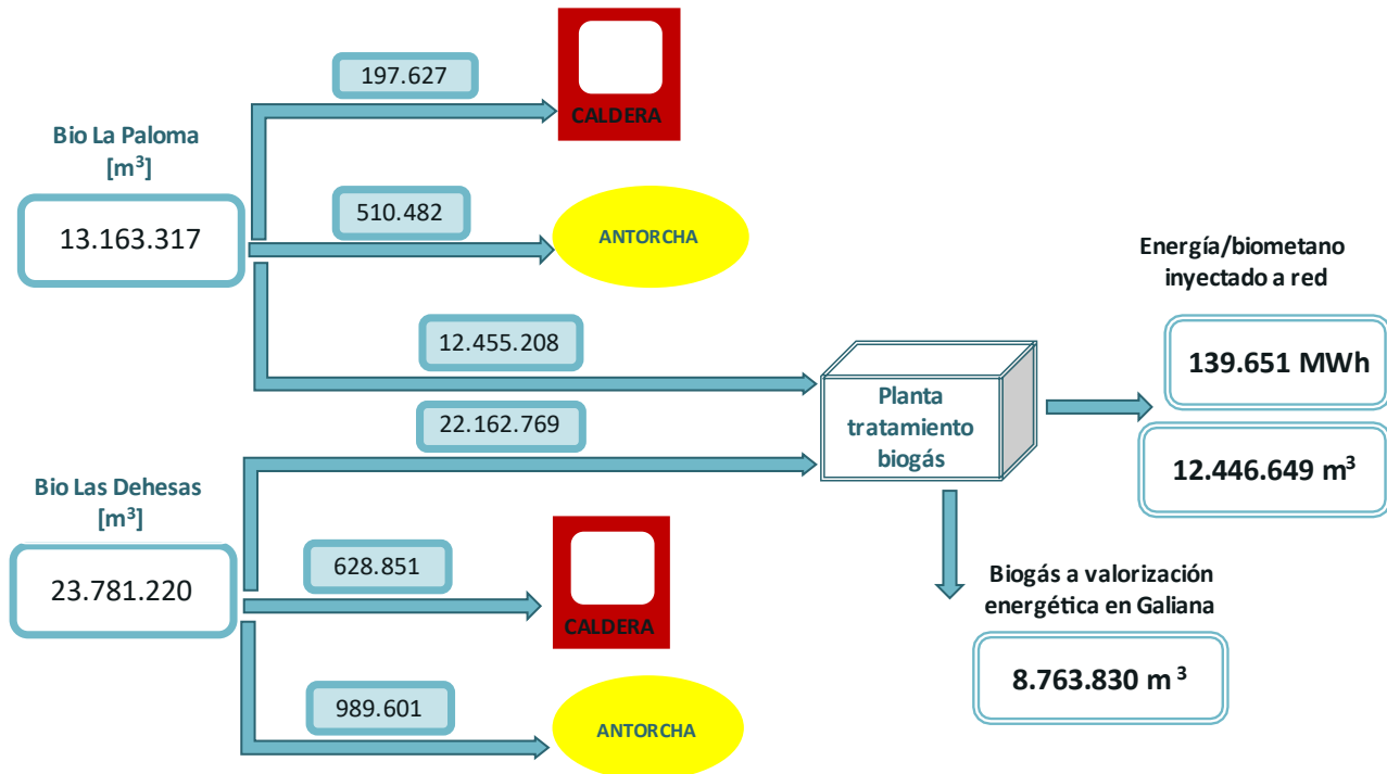
Gráfico 7.3. Producción de biogás y biometano en el complejo de biometanización, 2022
