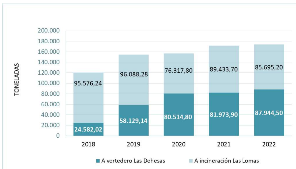
Gráfico 3.4. Destino de los rechazos generados en el centro La Paloma (2018-2022)
