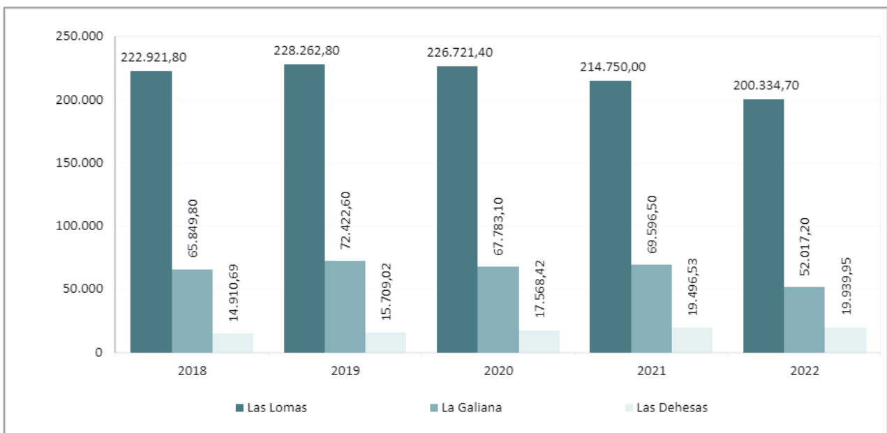
Gráfico 1.8. Origen de la electricidad generada (MWh) en el PTV (2018-2022)
