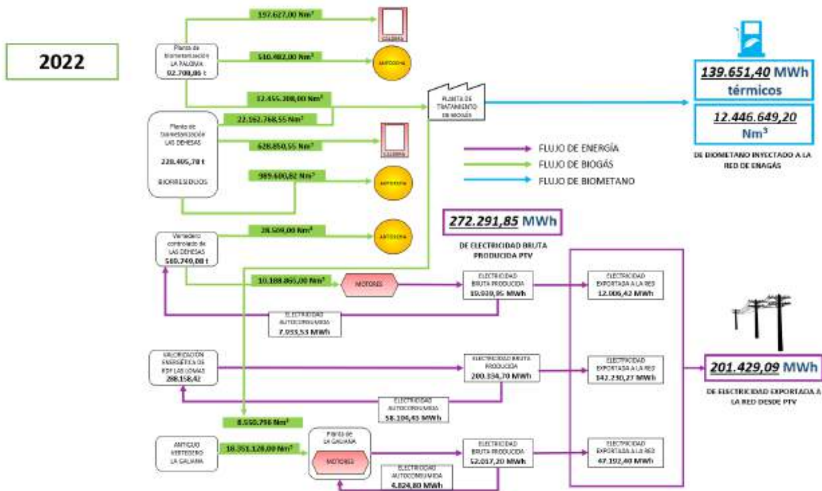
Gráfico 1.11. Principales flujos de biogás y energía del PTV (2022)
